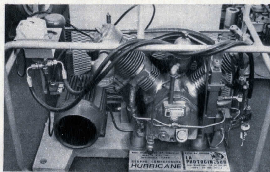
Sopra: il nuovo compressore americano "Hurricane E" elettrico ed a scoppio, carica a 225 atmosfere 2 gruppi di bombole nel tempo di 15 minuti.
