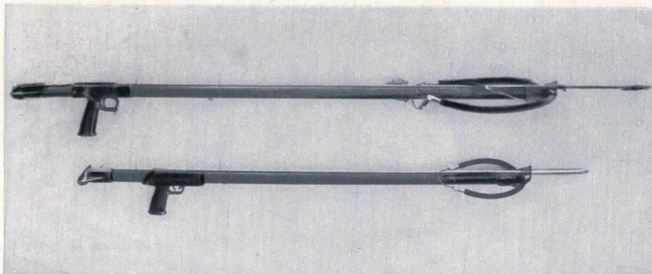
Il nuovo fucile oleopneumatico presentato dalla Technisub: a due potenze, canna schiacciata e calcio regolabile. Sotto: due Arbaletes ad elastici australiani importati dalla Salvas.
