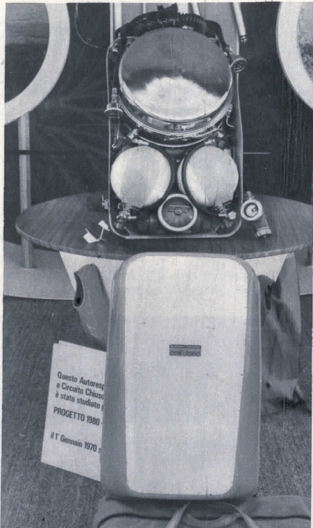
Il nuovo autorespiratore a circuito chiuso Back-Pack presentato dalla GSD: funzionante con miscela elio-ossigeno consente immersioni che raggiungono i 300 metri.
