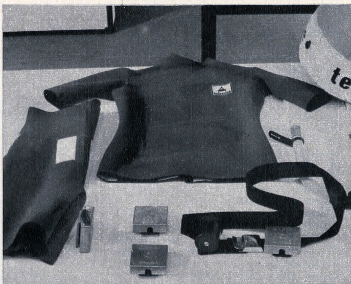
Della Technisub i nuovi pesi con piombi da 1 chilo ad innesto rapido e muta con maniche e calzoni corti in due pezzi.
