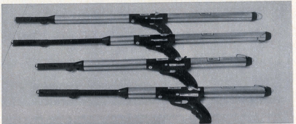
Sotto: la gamma completa dei fucili oleopneumatici presentati da Tecnisport in differenti lunghezze e potenze; dall'alto: il Makò, il Diabolo, il Vulcan e il Mirage.
