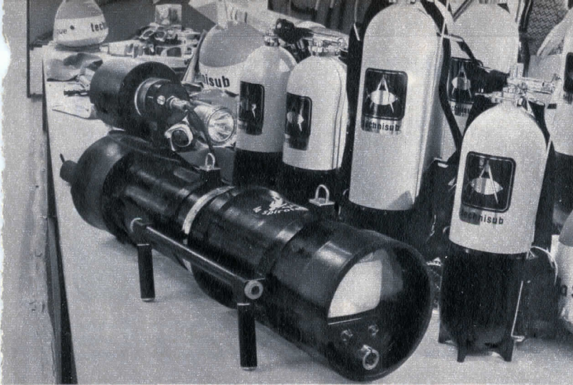
Una nuova telecamera subacquea presentata dalla Technisub e costruita da La Spirotechnique e la serie degli autorespiratori mono e bibombola dalle capacità variabili da 10 a 12 litri.
