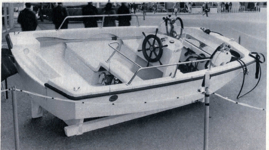
Sotto: la Salvias ha presentato il "Tiger Shark I" trimarano in fibra di vetro, la vera barca del sub: dispone infatti di un piccolo compressore che alimenta due narghilè posti a prua dell'imbarcazione e particolarmente utili per la decompressione. Ben studiate le sistemazioni interne per collocare i bibombola, fucili ed attrezzature varie.
