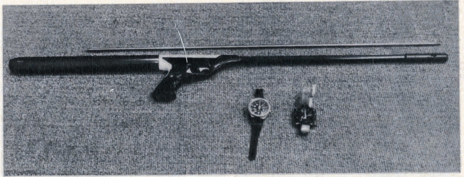
Il nuovo fucile "Dinamic" presentato dalla GSD: oleopneumatico a due potenze regolabili insieme ad un altro accessorio: il profondimetro con scala graduata fino a 120 m.
