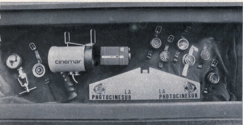
Nella foto sotto: la custodia subacquea Cinemar della Photocinesub, per la cinepresa Super 8 automatica elettrica Kodak M 14; tutta la serie di profondimetri, bussole e manometri.
